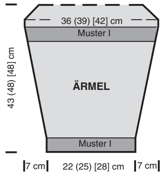
SCHNITTÜBERSICHT
